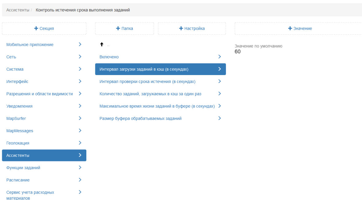
Рис. 2.261: Интервал загрузки заданий в кэш
