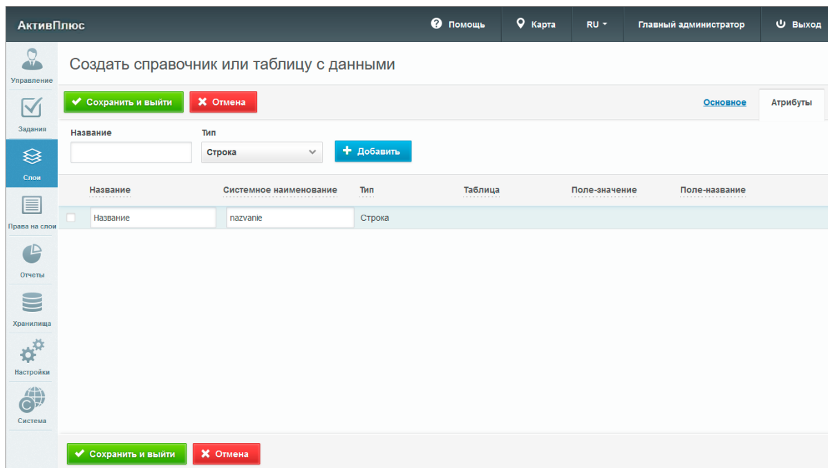
Рис. 2.84: Добавление атрибутивных данных таблицы
