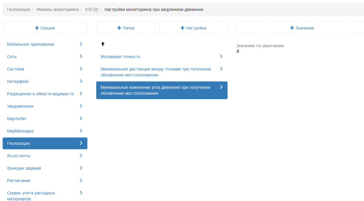
Рис. 2.239: Минимальное изменение угла движения
