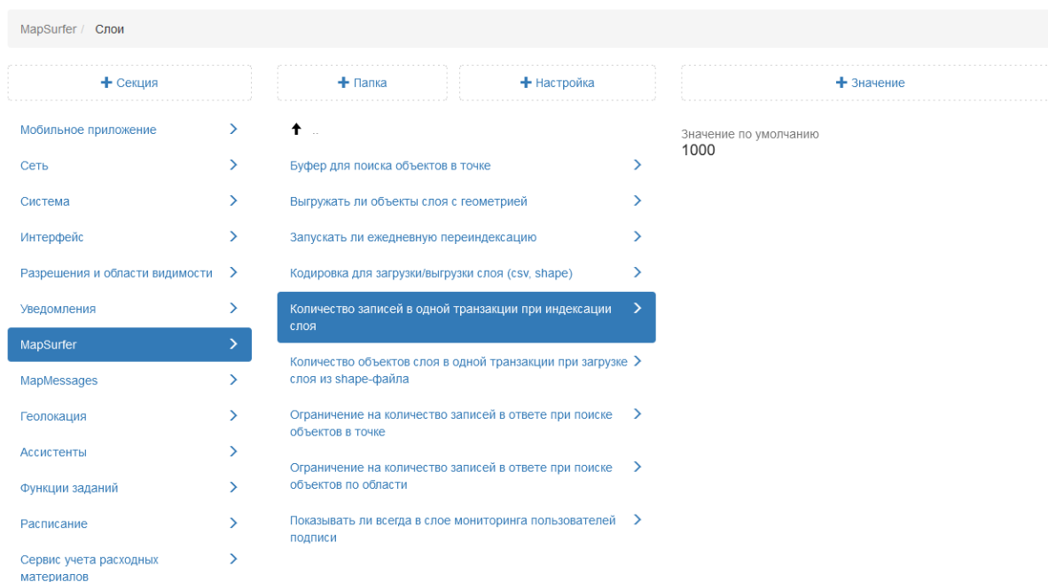
Рис. 2.214: Количество объектов слоя в одной транзакции при загрузке слоя из share-файла
