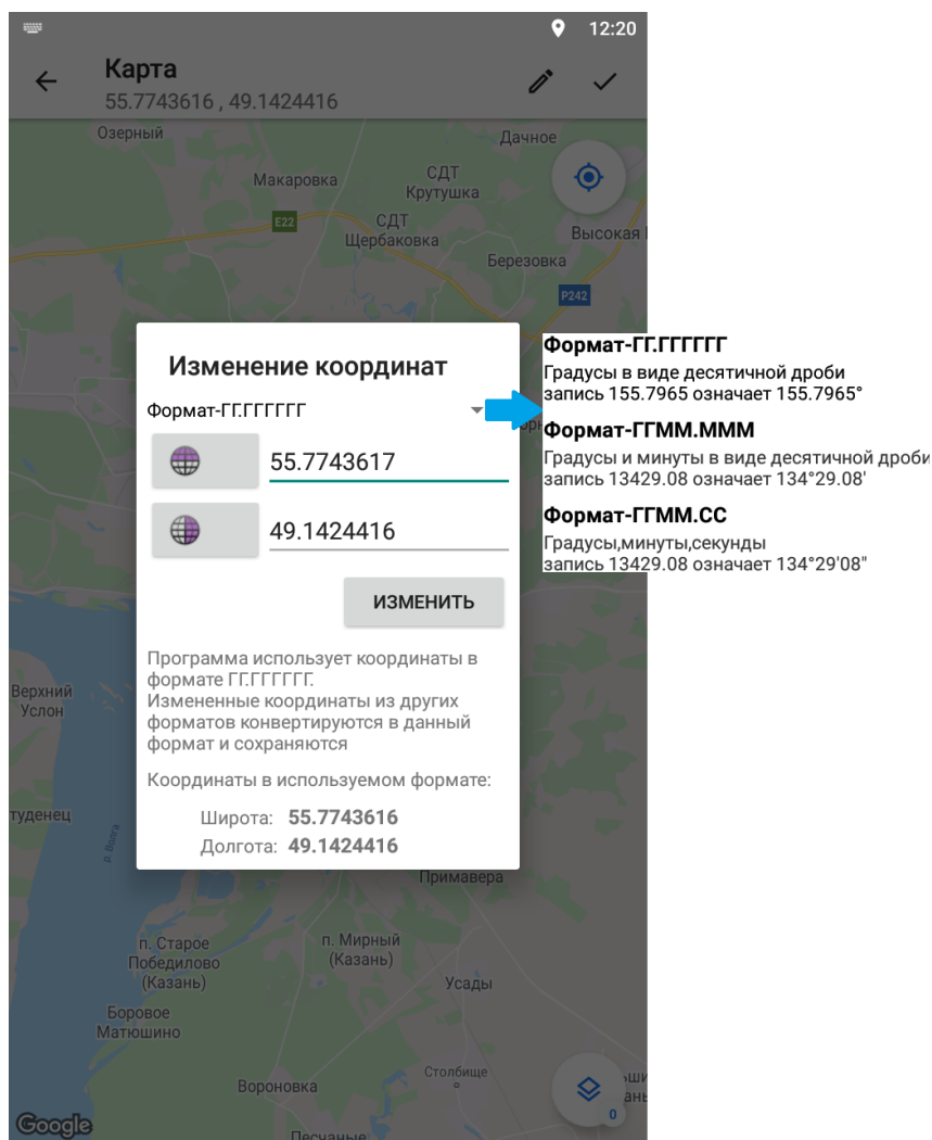
Рис. 2.30: Изменение координат
