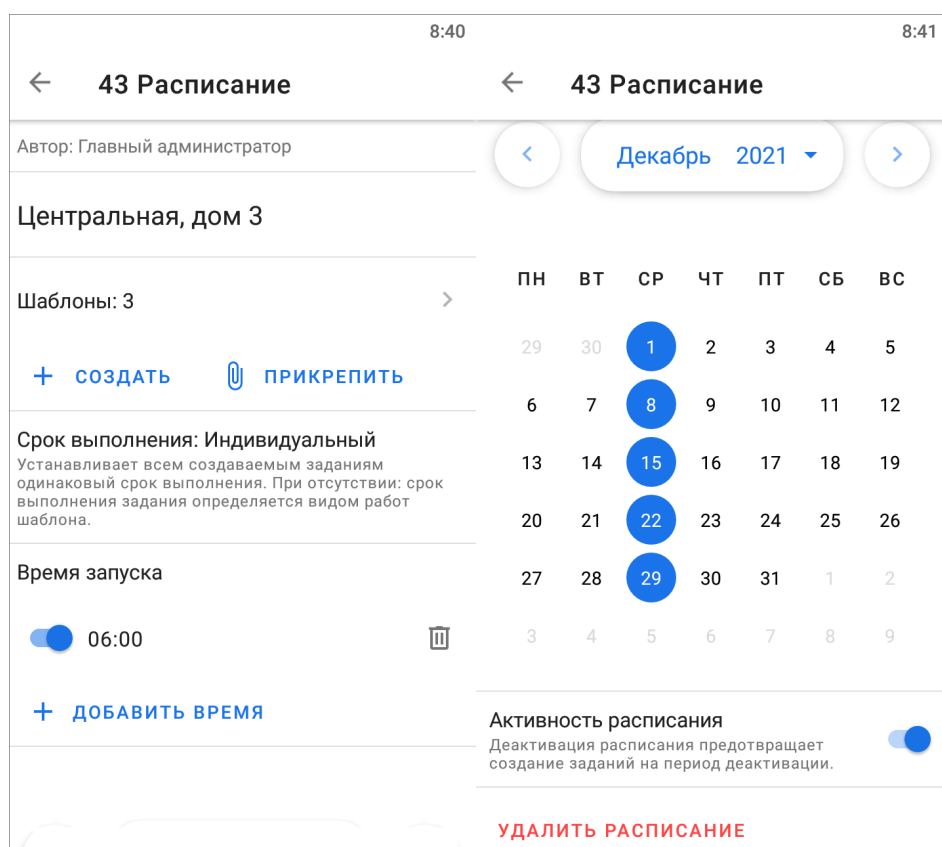
Рис. 2.68: Создание расписания
