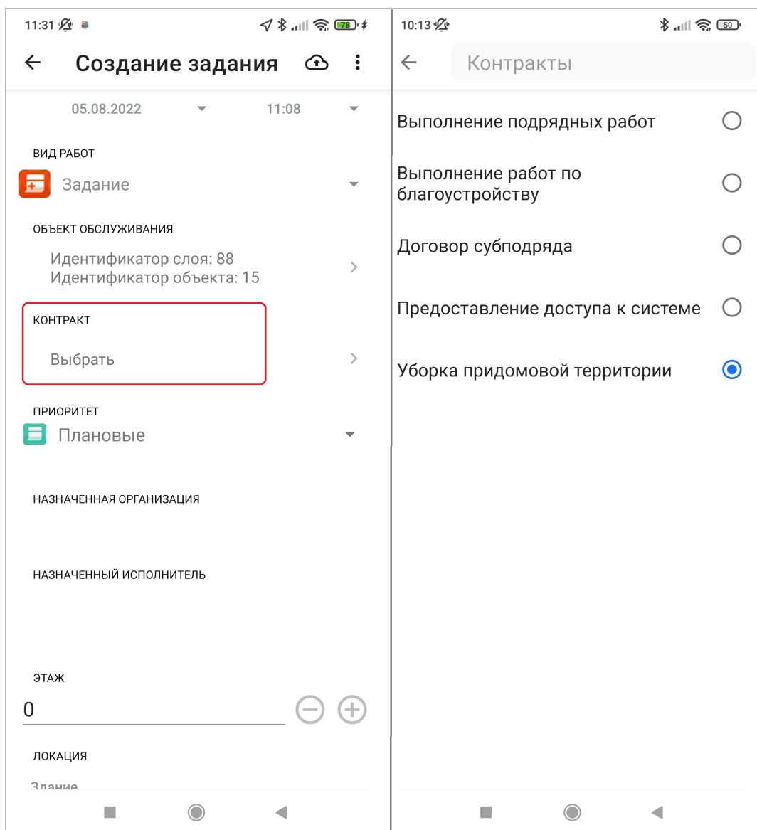
Рис. 2.27: Прикрепление контракта
