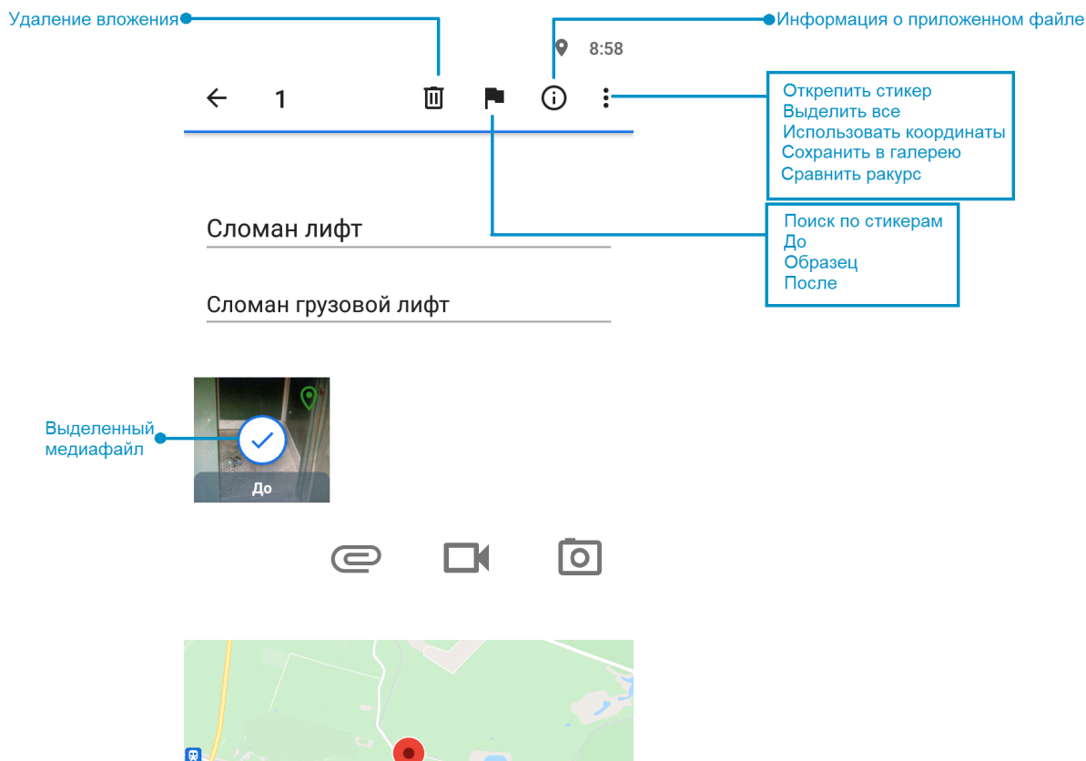
Рис. 2.21: Схема окна «Создания задания» в режиме работы с медиафайлами
