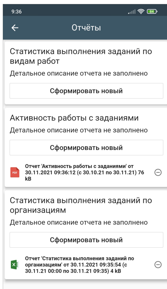
Рис. 2.71: Окно «Отчеты»
