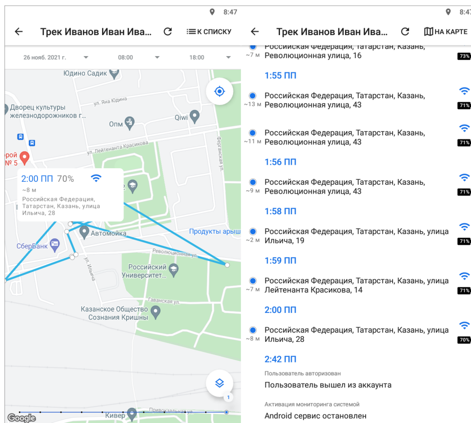
Рис. 2.62: Просмотр трека
