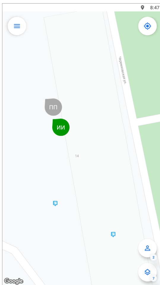
Рис. 2.56: Окно «Карта»
