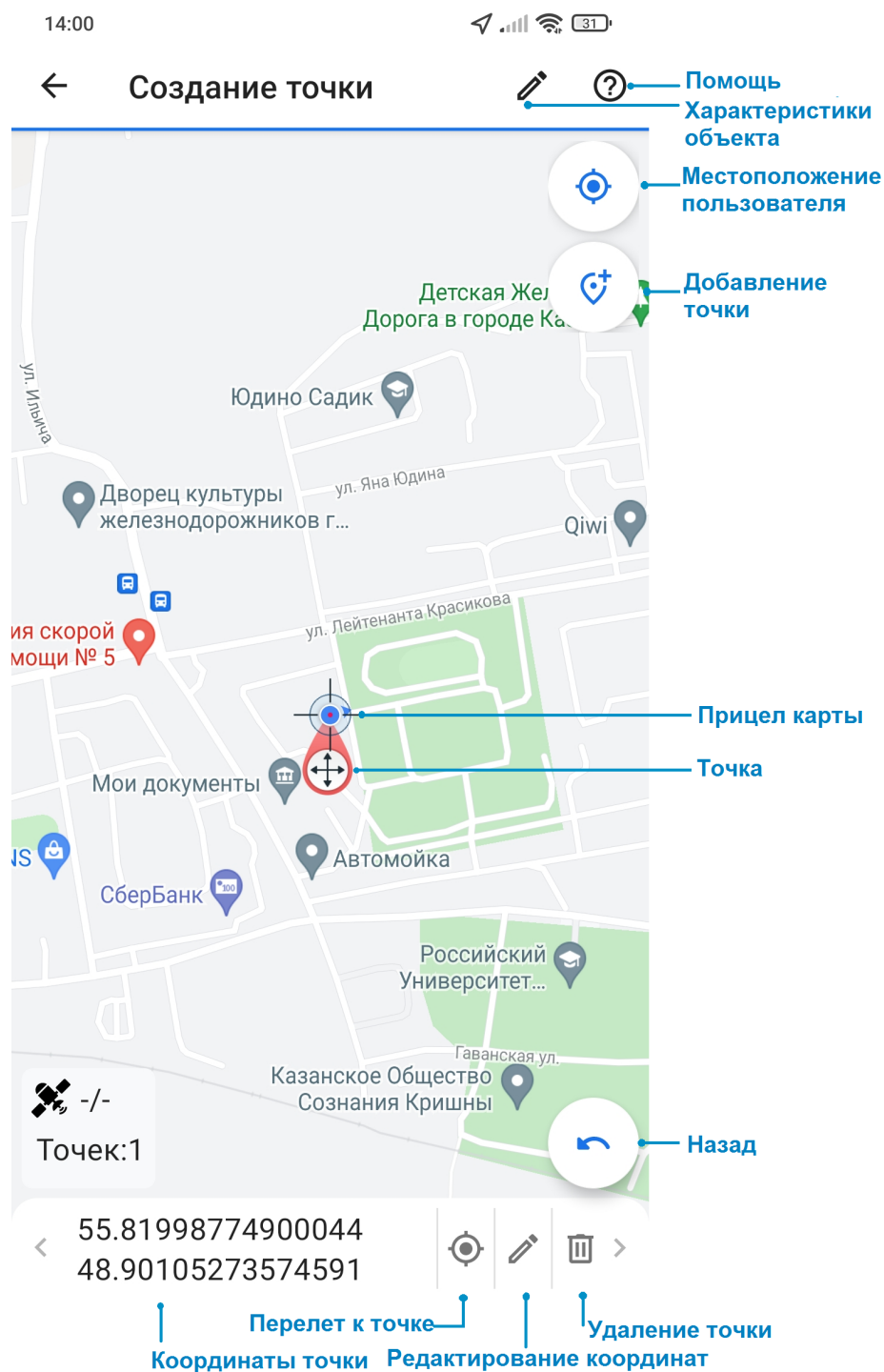
Рис. 2.46: Окно добавления точечных объектов
